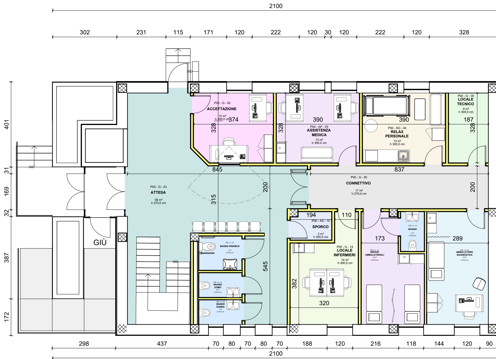
DISTRIBUZIONE FUNZIONALE PIANO TERRA SCALA 1:100
